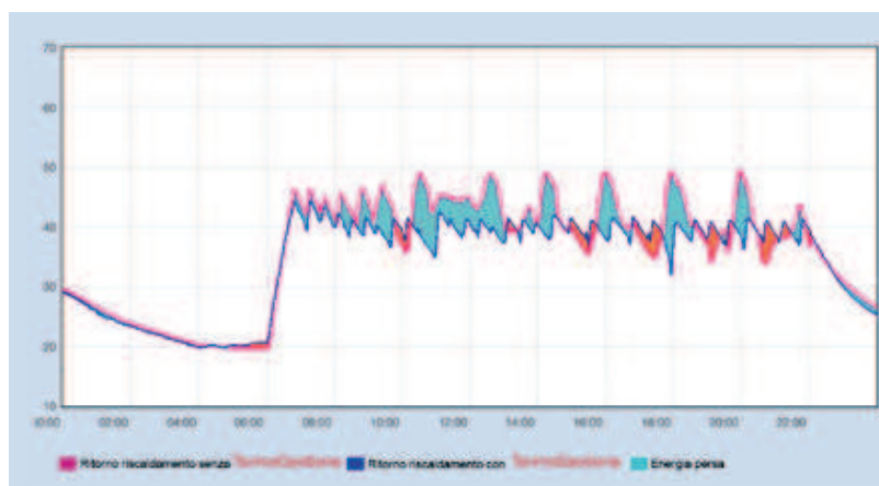
Immagine 6 Sovrapposizione dei precedenti grafici per individuazione minor energia ceduta (differenza grafici sui soli ritorni impianto)
