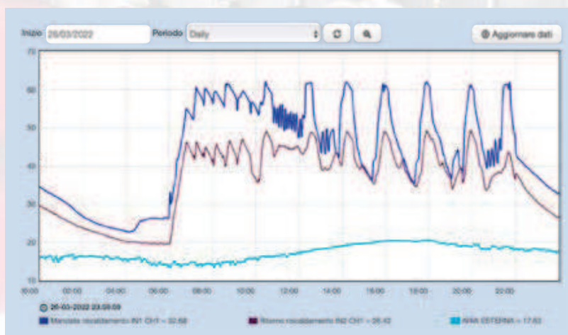
Immagine 4 Andamento temperature mandata (blu) e ritorno (marrone) dell'impianto campione senza ottimizzazione
